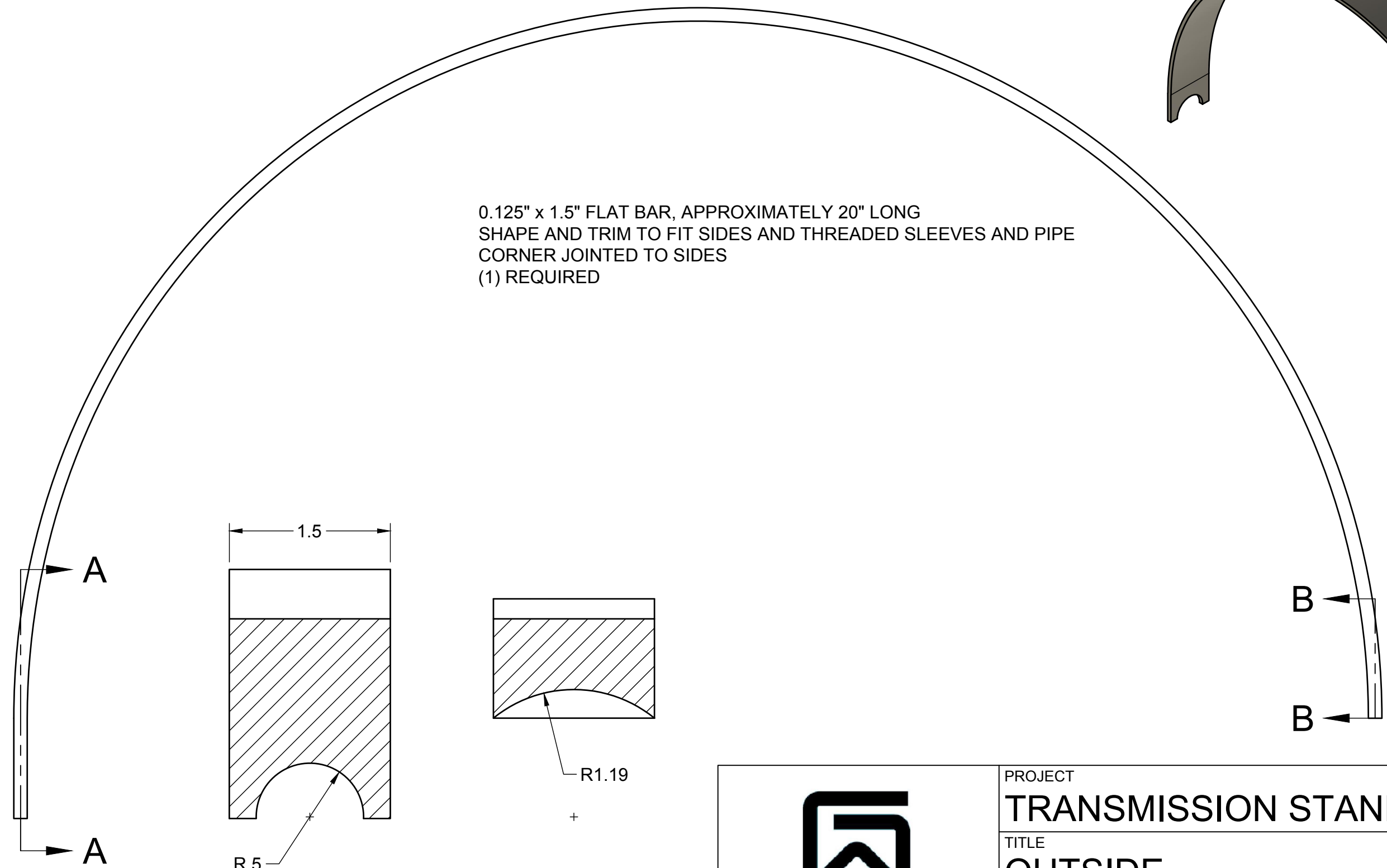
SECTION A-A SCALE 1:1
